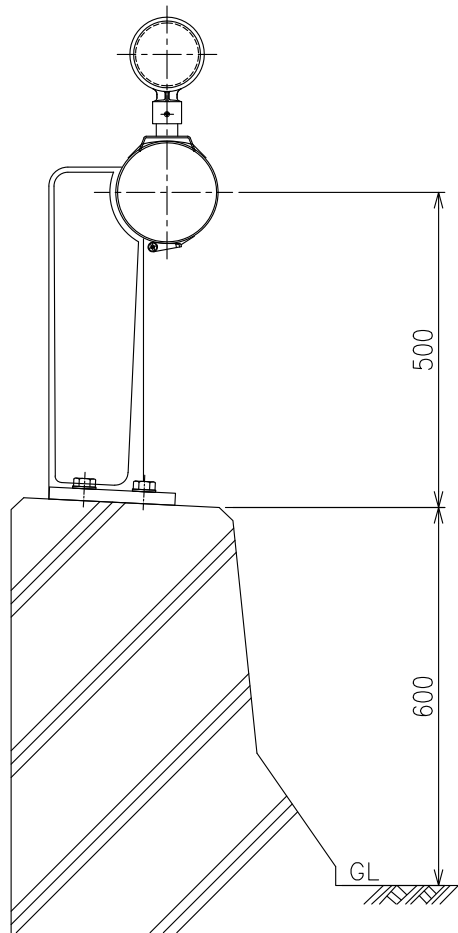
設置図 S=1:12
